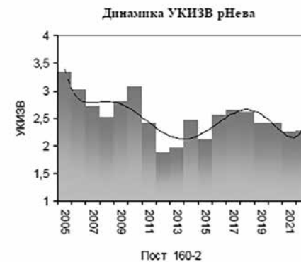
Рис. 5.4. Многолетняя динамика УКИЗВ. р. Нева, створ 2
