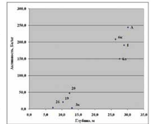
Рис. 5.28. Средние значения удельной активности \text{Cs-137} в пробах донных отложений по результатам исследований 2016-2022 гг. в зависимости от глубины отбора
