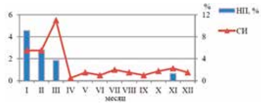
Рис. 7.3. Годовой ход значений СИ и НП сероводорода, г. Светогорск, 2022
