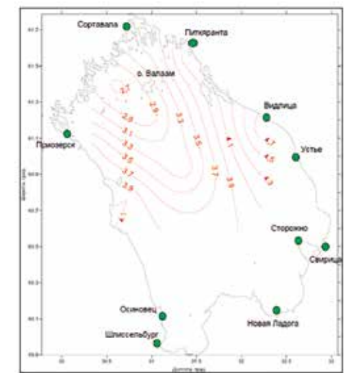
Рис. 5.14. Распределение температуры воды (°С) на глубине 30 м. Ладожское озеро, 29 мая – 01 июня 2022 года
