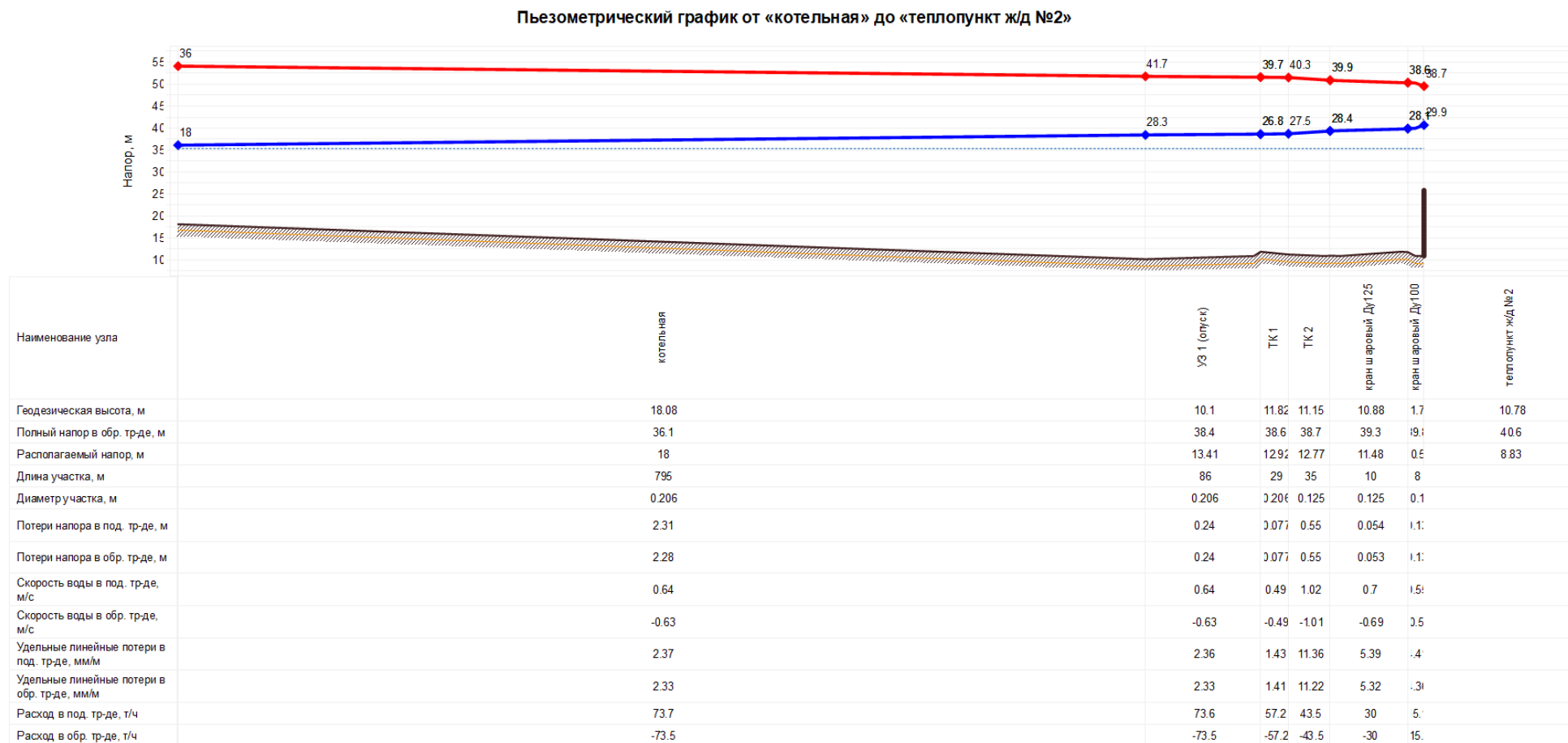
Рисунок 1.6 Пьезометрический график от котельной до индивидуального теплового пункта жилого дома (ул. Новая, 2) (фактический режим работы тепловых сетей)
