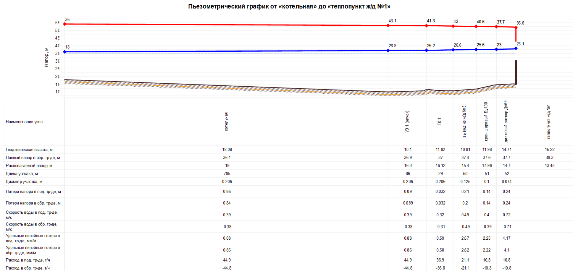
Рисунок 1.10 Пьезометрический график от котельной до индивидуального теплового пункта жилого дома (ул. Новая, 1) (с учетом выполнения наладочных работ)
