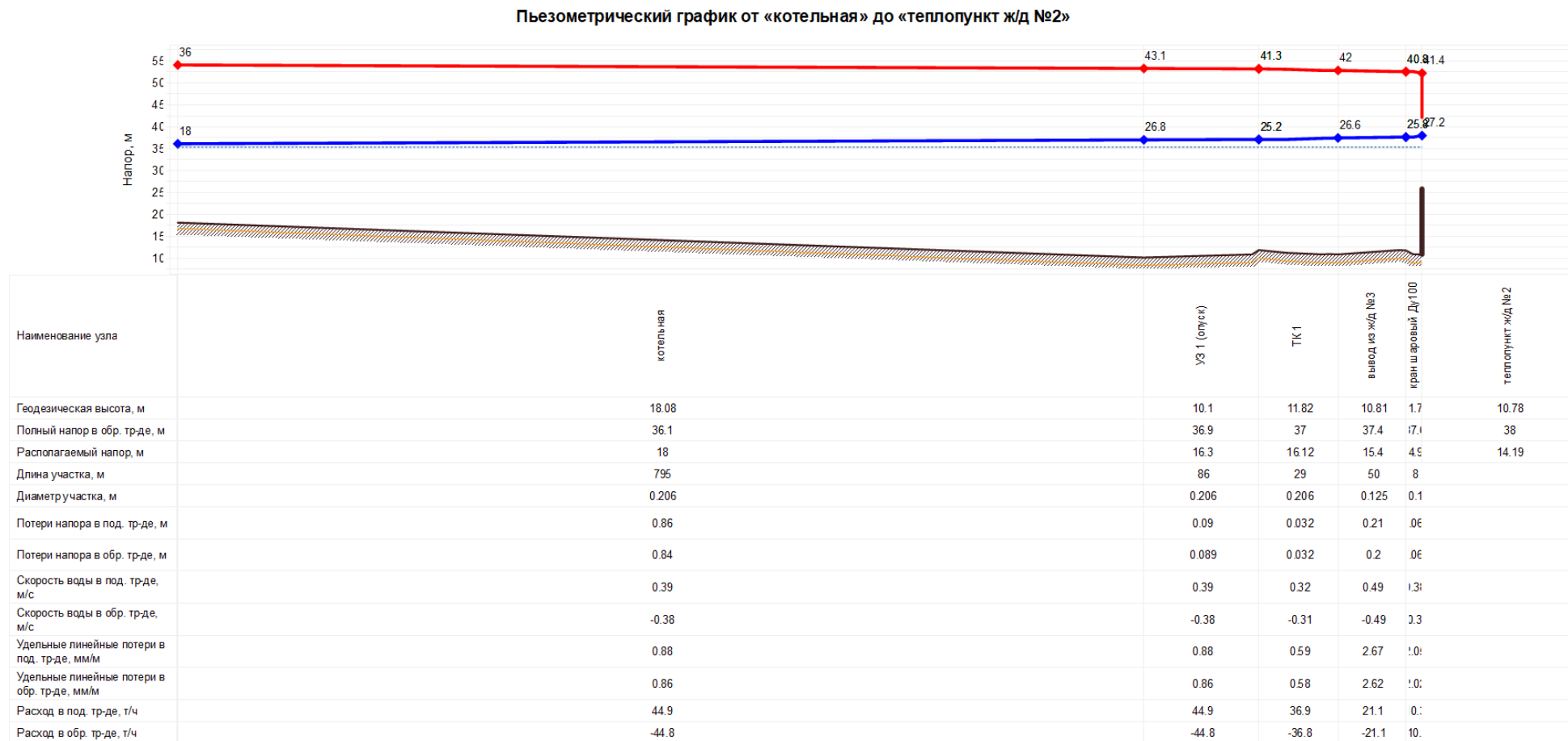
Рисунок 1.9 Пьезометрический график от котельной до индивидуального теплового пункта жилого дома (ул. Новая, 2) (с учетом выполнения наладочных работ)
