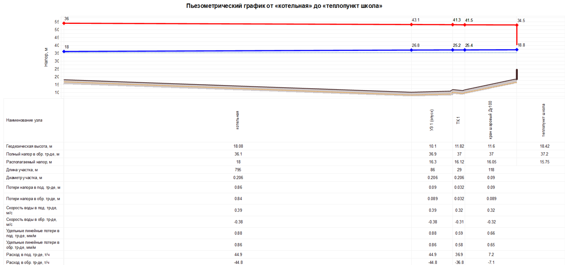
Рисунок 1.8 Пьезометрический график от котельной до индивидуального теплового пункта школы (с учетом выполнения наладочных работ)
