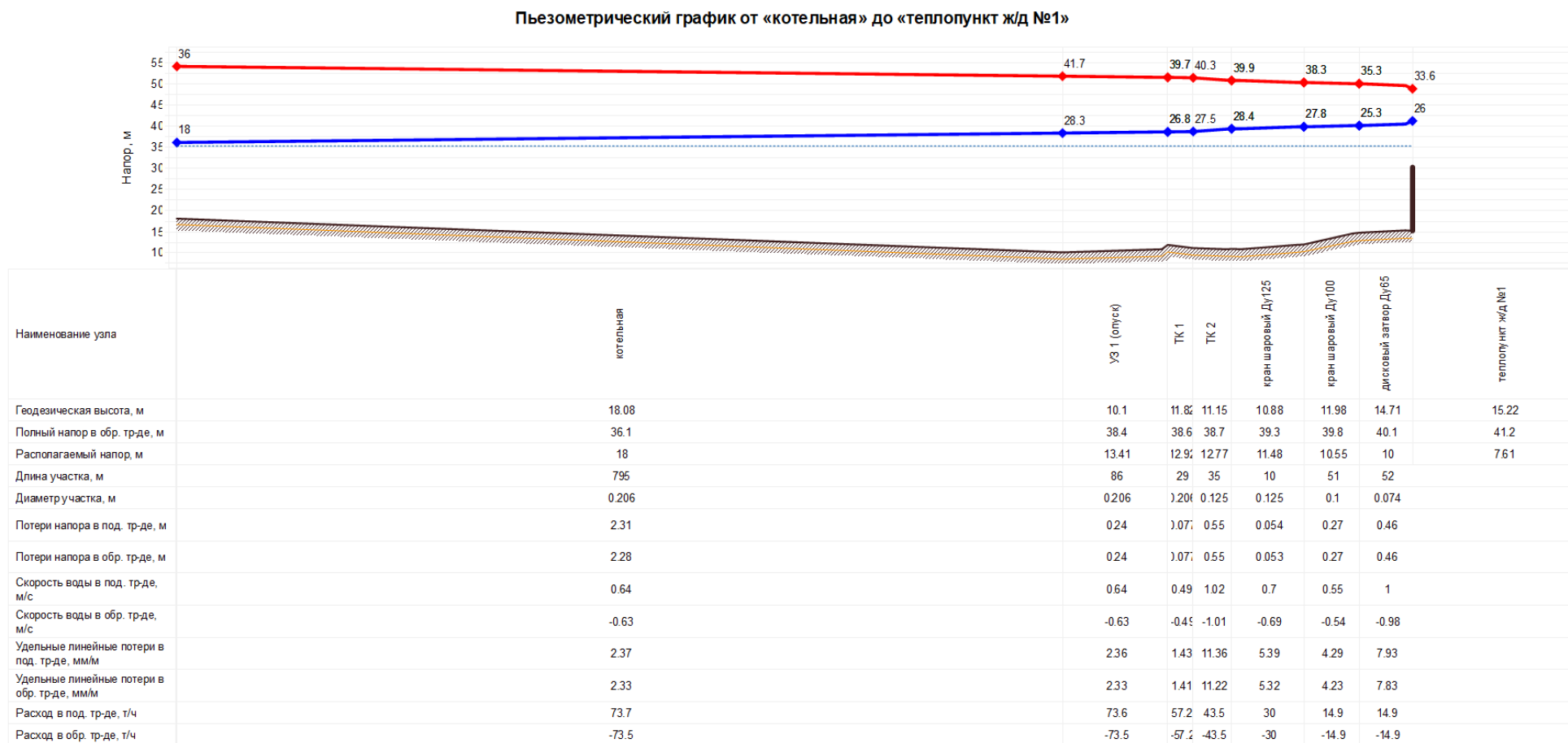
Рисунок 1.7 Пьезометрический график от котельной до индивидуального теплового пункта жилого дома (ул. Новая, 1) (фактический режим работы тепловых сетей)
